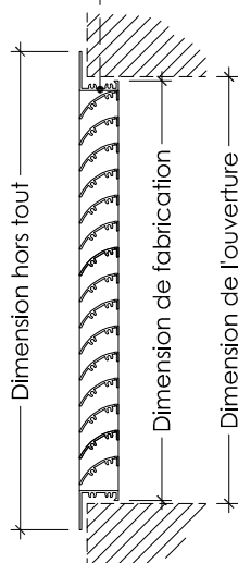
Cadre en "L" (CL)
