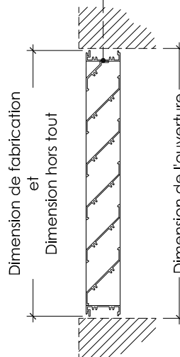
Cadre en "U" (CU)
