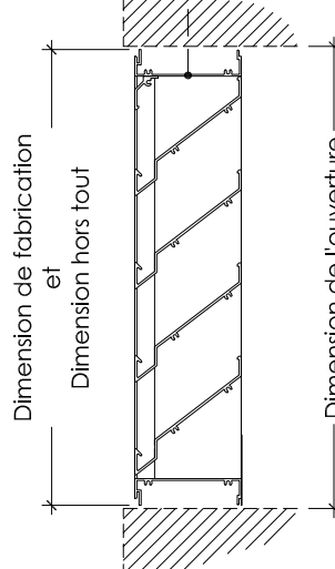
Cadre en "U" (CU)
