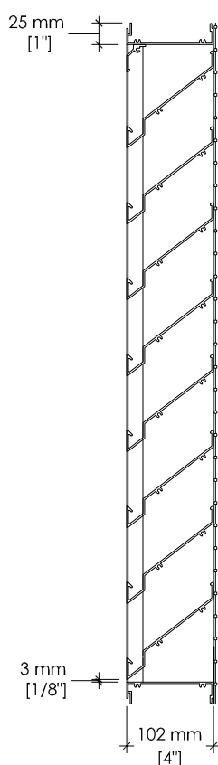
Cadre en "U" (CU)
