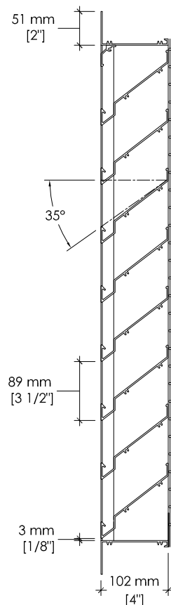
Cadre en "L" (CL)
