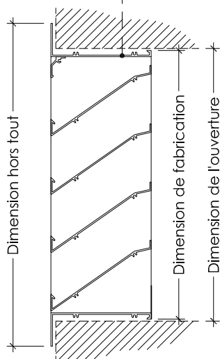
Cadre en "L" (CL)
