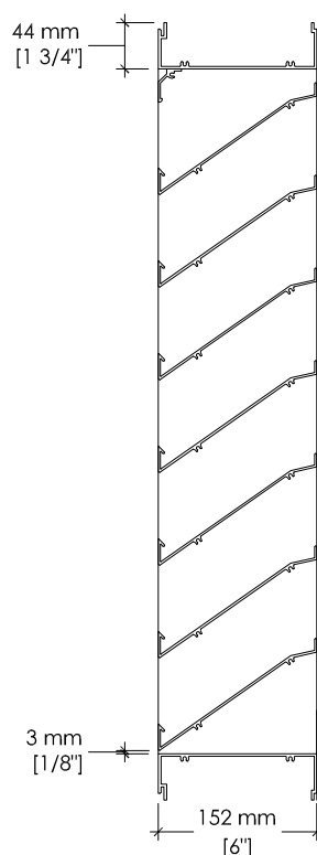
Cadre en "U" (CU)
