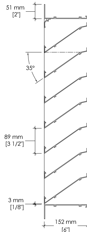
Cadre en "L" (CL)
