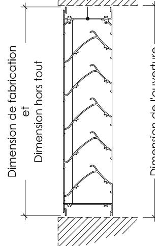
Cadre en "U" (CU)
