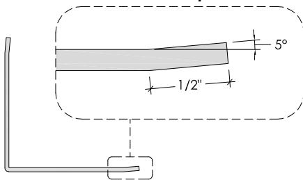
Détail du repli de 5°
