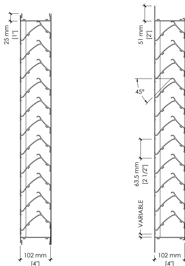
Cadre en "U" (CU)
