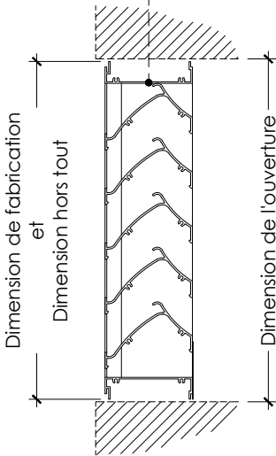
Cadre en "U" (CU)
