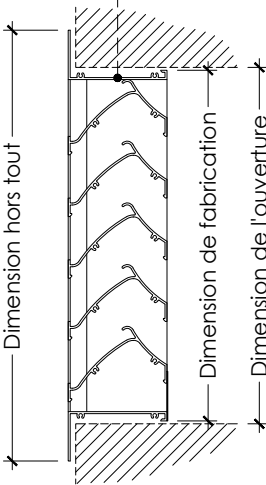
Cadre en "L" (CL)
